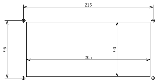
パネルカット寸法詳細図 尺度：1/2
